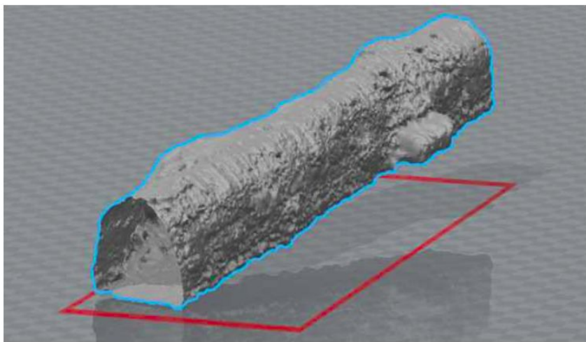
Exemplo de modelo 3D de túnel de adução
